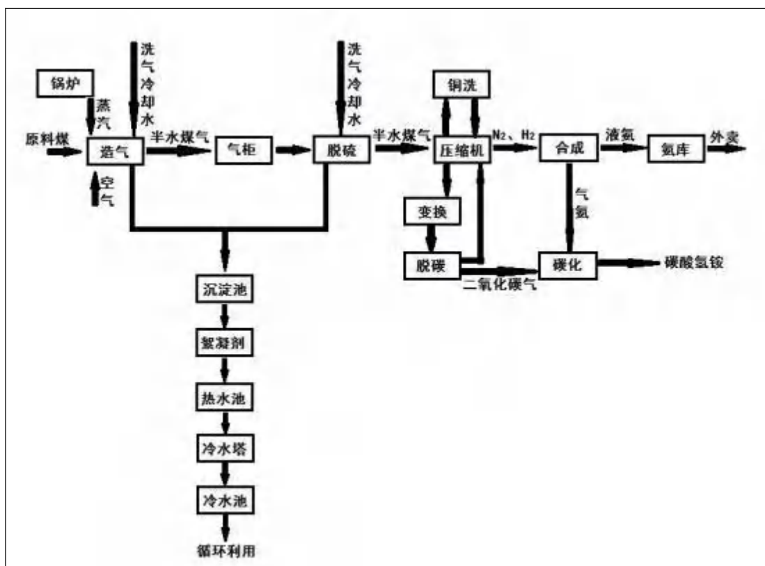
图 3-16 合成氨—联产碳酸氢铵生产工艺流程
