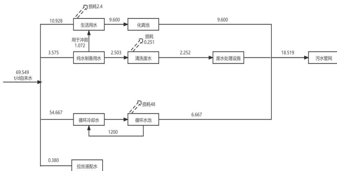
图 3.6-1 项目水平衡图 单位：t/d
