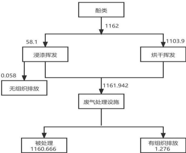
图 3.5-3 项目油漆酚类平衡图 单位：t/a
