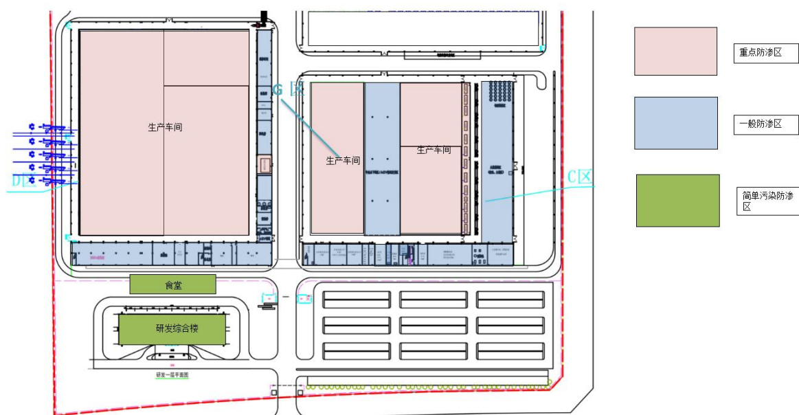
图 4.2-1 厂区分区防渗图
