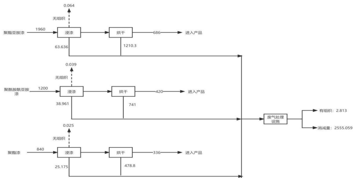
图 3.5-1 项目 VOC 平衡图 单位：t/a
