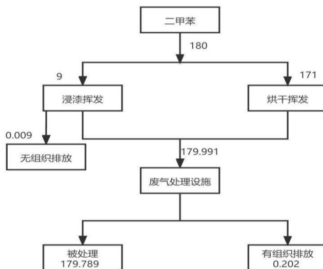
图 3.5-2 项目油漆二甲苯平衡图 单位：t/a
