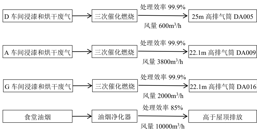
图 4.1.2-1 废气处理工艺流程图
