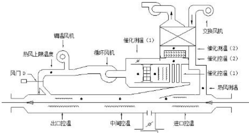
图 4.1.2-2 漆包机催化燃烧处理有害气体原理图
