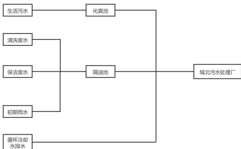
图 4.1.1-1 废水处理措施流程图
