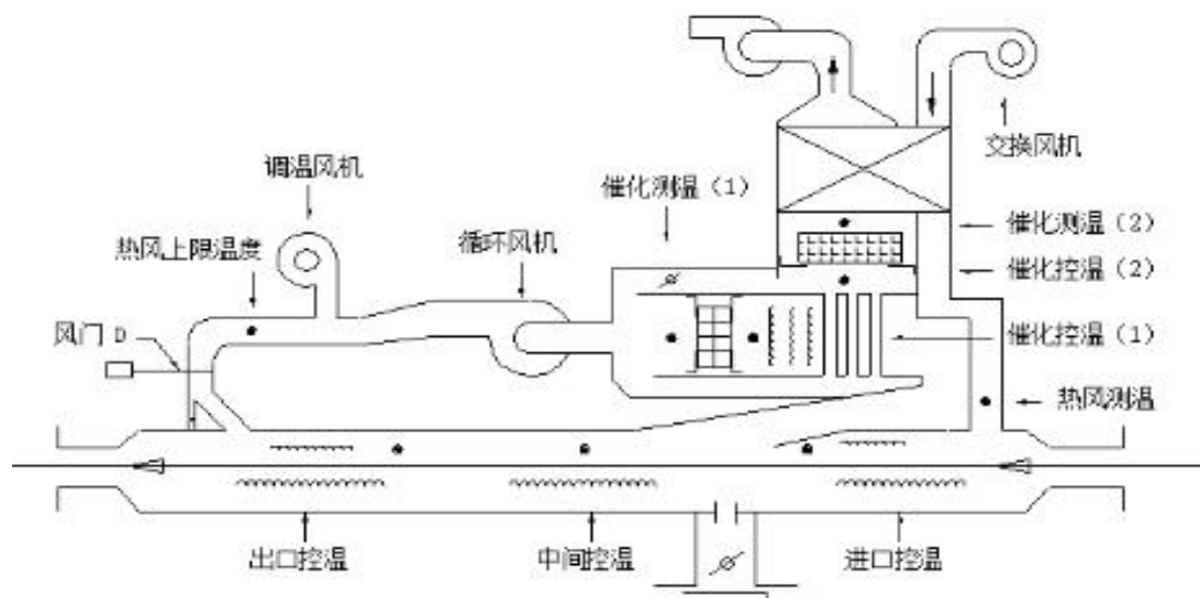
图 4.1.2-2 漆包机催化燃烧处理有害气体原理图
