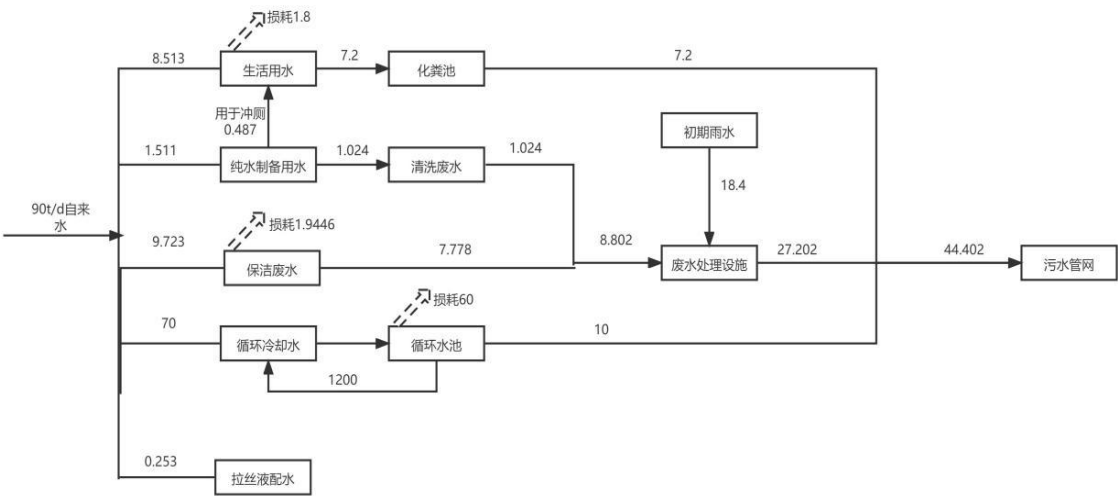
图 3.6-1 项目水平衡图 单位：t/d
