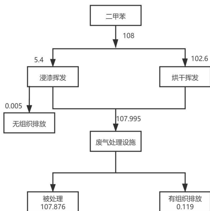
图 3.5-2 项目油漆二甲苯平衡图 单位：t/a
