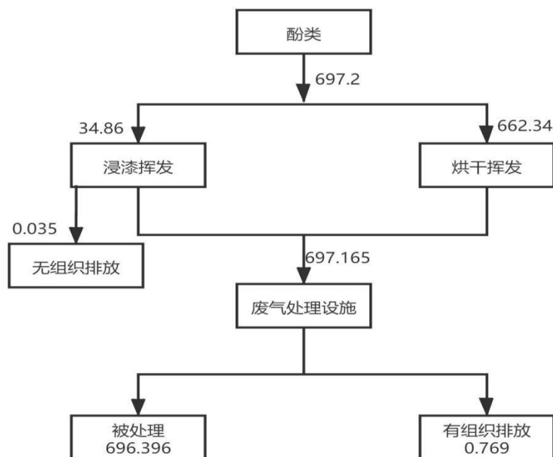
图 3.5-3 项目油漆酚类平衡图 单位：t/a
